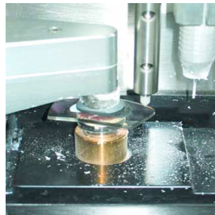
Sistema robotizzato di foratura glasant
